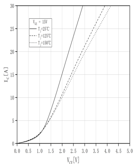
输出特性 IGBT, 制动—斩波器 (典型) output characteristic IGBT, Brake-chopper (typical) V_{GE} = 15V
