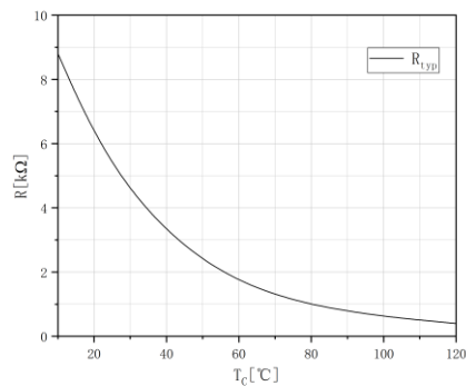
NTC 温度曲线 (典型) NTC Temperature Characteristics
