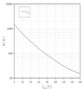
负温度系数热敏电阻温度特性 (典型) NTC-Thermistor-temperature characteristic (typical)
